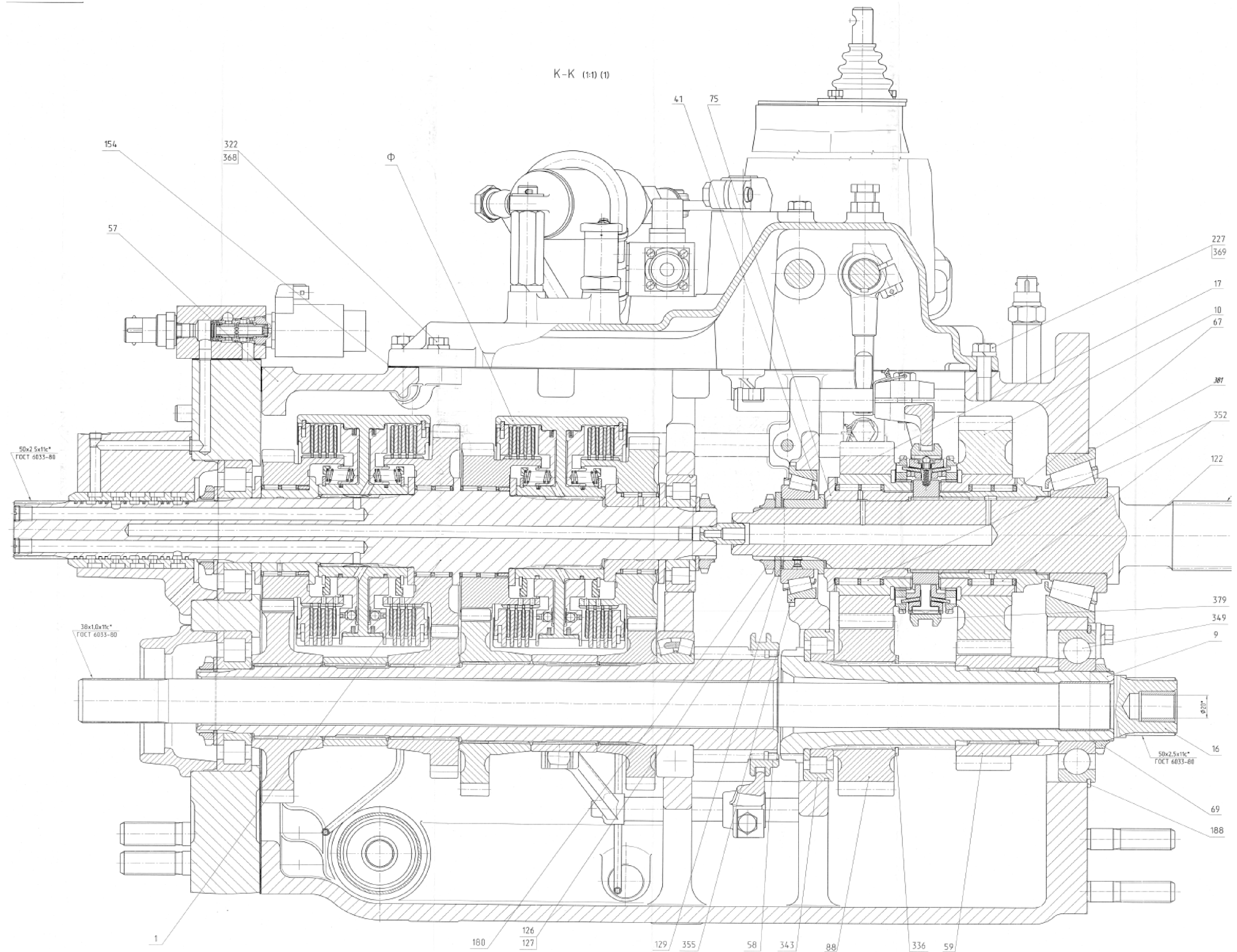
Рисунок 1 (лист 7 из 7) - Коробка передач
