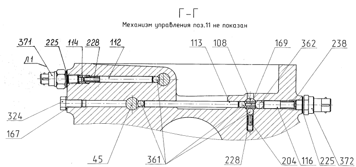
Рисунок 1 (лист 1 из 7) – Коробка передач.
