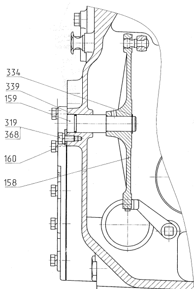
Рисунок 1 (лист 6 из 7) – Коробка передач.
