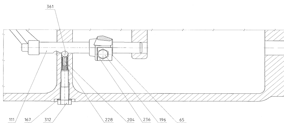
Рисунок 1 (лист 4 из 7) – Коробка передач.
