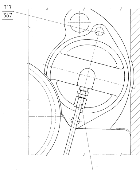
Рисунок 1 (лист 6 из 7) – Коробка передач.
